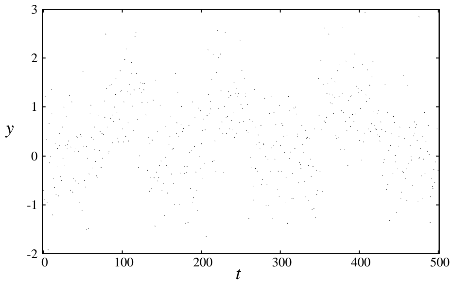
図 4: 観測値 y_t
